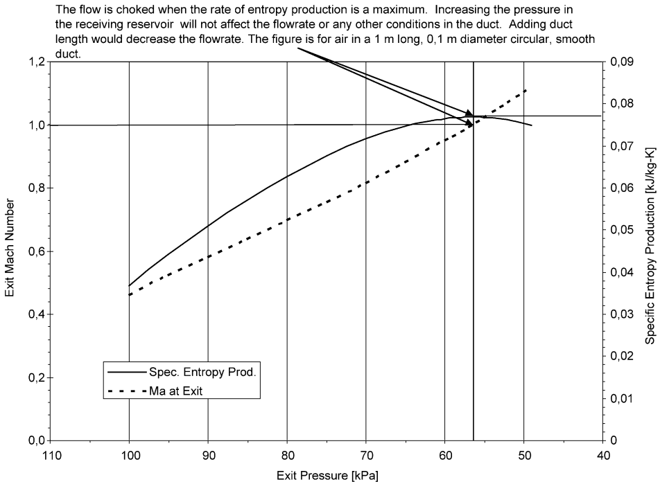
Fig. 5. Fanno flow example.
